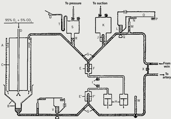
Circuito extracorpóreo de membrana de Gibbon
