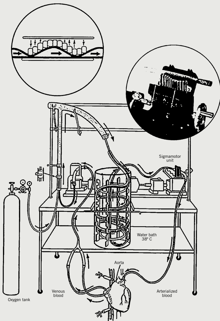
Diagrama de 1955 DeWall-Lillehei con depósito de hélice y oxigenador de burbuja desechable con capacidad para adultos. Destaca la columna de oxigenación en posición vertical con la mezcla de sangre venosa y burbujas de oxígeno formadas en la base. También destacar la cámara de eliminación de burbujas transversal, y la espiral (helicoidal) para eliminar las burbujas del depósito sumergido en un baño de agua. Los dos detalles muestran el patrón ondulatorio de 12 "dedos" de la bomba Sigmamotor metálicos, que permite acariciar la sangre a través del tubo de plástico sin contacto directo.
